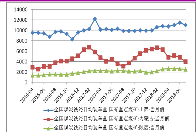
图 8: 全国煤炭铁路日均装车量 车/天
